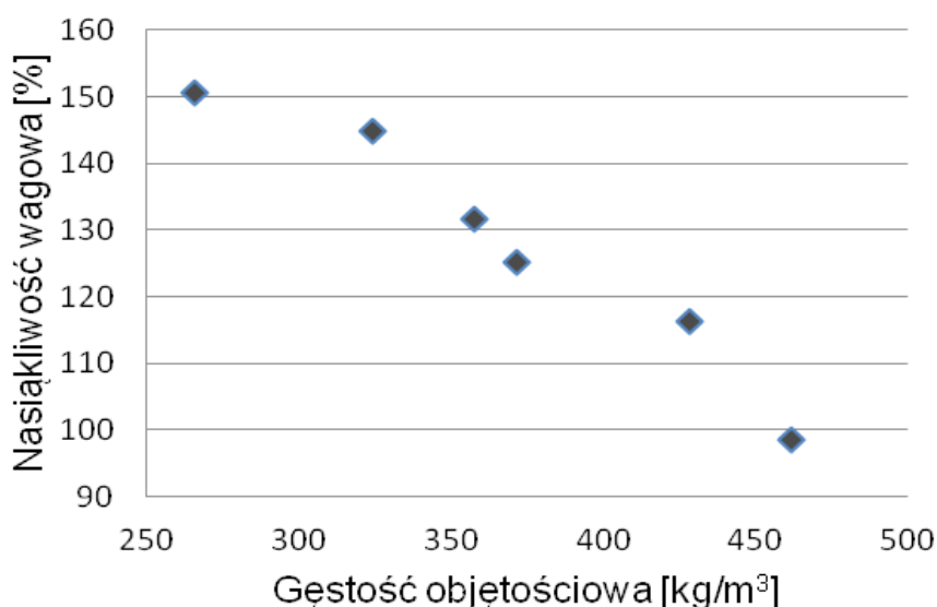
Figure 8. The dependency of thermal conductivity coefficient of the composite and its bulk density Rysunek 8. Zależność współczynnika przewodności cieplnej kompozytu od jego gęstości objętościowej Source: the authors' archive based on Barnat-Hunek et al. 2015, Barnat-Hunek et al. 2016. Źródło: archiwum autorów na podstawie Barnat-Hunek i in. 2015, Barnat-Hunek i in. 2016.
