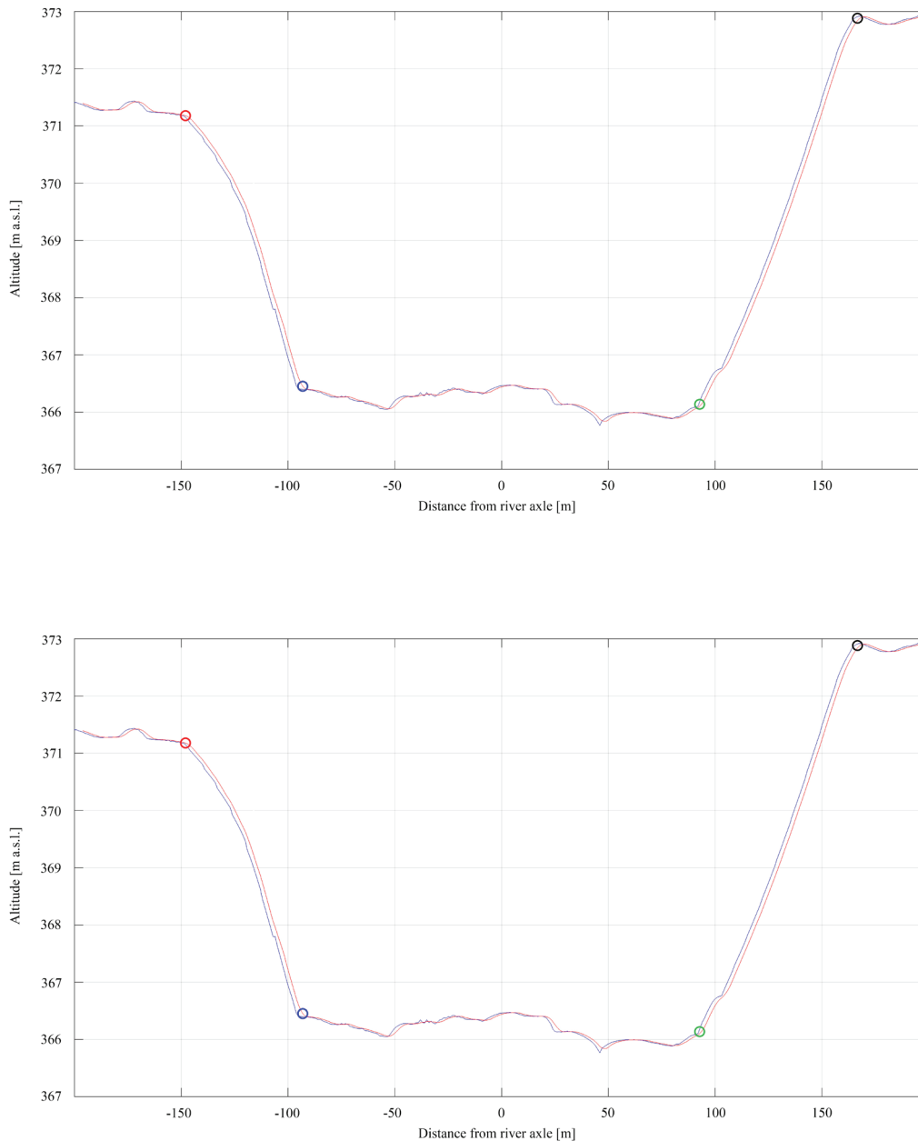
Figure 8. Procedure for the identification of the bottom and top of both riversides and the terrain profile for each transversal section previously identified. In a), the blue line represents the first derivative (slope) of the section, while the red one represents the moving average of the calculated first derivative. The black dashed line represents the thresholds used to detect the POIs: when the moving average of the derivate overpasses these thresholds, the POIs are set-up, identifying the top (POI1) and bottom (POI2) of the left riverside (red and blue circle) and the bottom (POI3) and top (POI4) of the right riverside (green and black circle). In b), the riverside terrain profile is reported. The blue line represents the actual height of the section, while the red line represents the moving average of the height of the section. Also, the four POIs are reported in this figure. Abbildung 8. Verfahren zur Identifizierung der Unter- und Oberseite beider Flussufer und des Geländes für jeden zuvor identifizierten Querschnitt. In a) repräsentiert die blaue Linie die erste Ableitung (Steigung) des Abschnitts, während die rote den gleitenden Durchschnitt der berechneten ersten Ableitung darstellt. Die schwarze gestrichelte Linie stellt die Schwellwerte dar, die zum Ermitteln der POIs verwendet werden: Wenn der gleitende Durchschnitt der Ableitung diese Schwellwerte überschreitet, werden die POIs eingerichtet, die den oberen (POI1) und unteren (POI2) Bereich des linken Flussufers (roter und blauer Kreis) sowie die Unterseite (POI3) und die Oberseite (POI4) des rechten Flussufers (grüner und schwarzer Kreis) identifizieren. In b) wird das Profil des Flussgeländes dargestellt. Die blaue Linie stellt die tatsächliche Höhe des Abschnitts dar, während die rote Linie den gleitenden Durchschnitt der Höhe des Abschnitts abbildet. In dieser Abbildung sind auch die vier POIs eingezeichnet.
