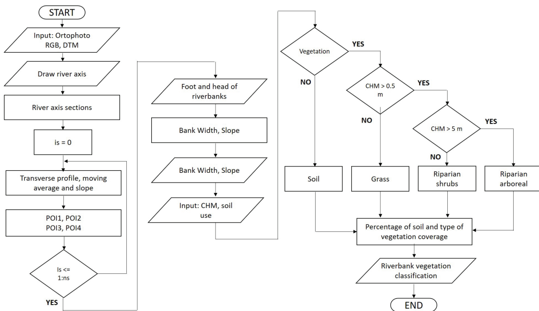
Figure 5. Flow-chart of the algorithm for riverbanks identification and the classification of the riparian strip vegetation. Abbildung 5. Flow-Chart des Algorithmus zur Identifizierung des Ufers und der Klassifizierung des Bodens und der Ufervegetation.
