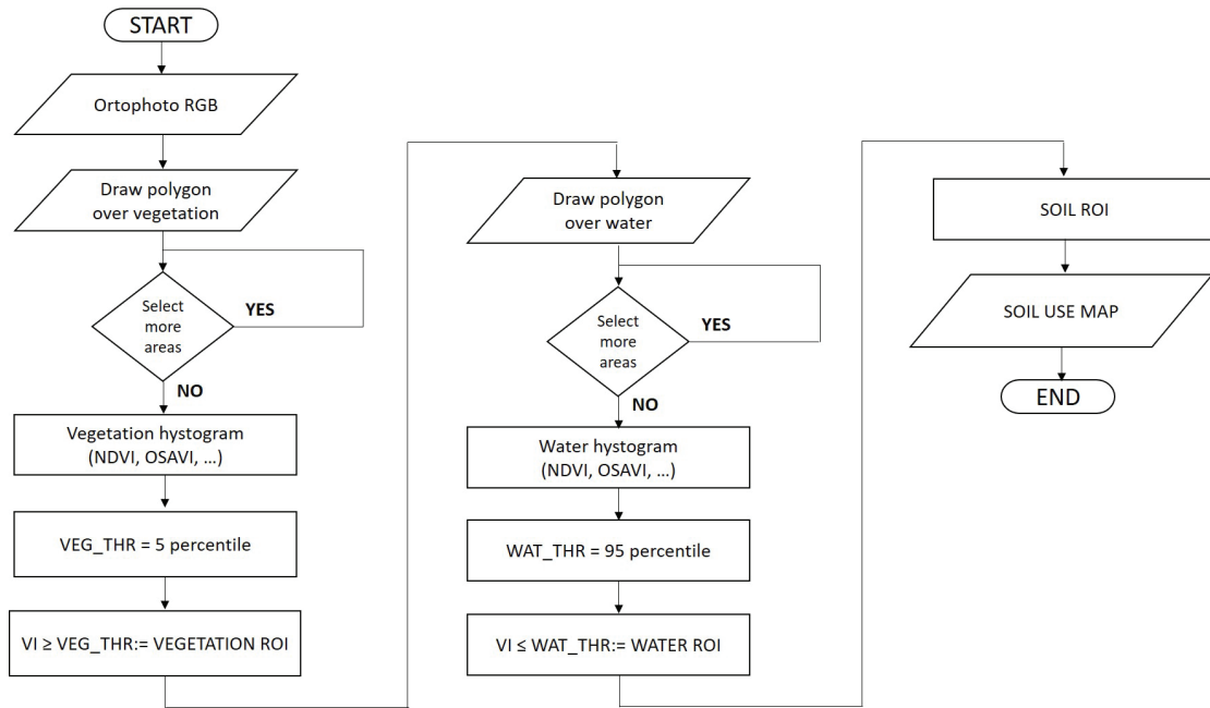
Figure 2. Land use algorithm flow-chart. Abbildung 2. Flow-Chart des Bodennutzungsalgorithmuses.
