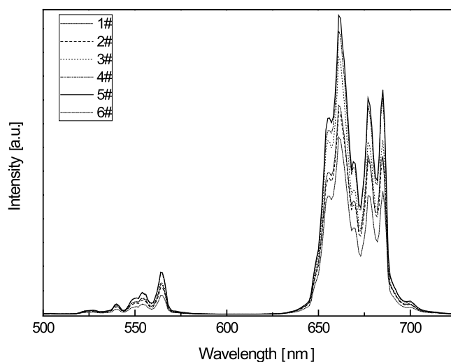
Figure 2. UC emission spectra of \text{Yb}^{3+} / \text{Er}^{3+} /GZO ceramics under 980 nm excitation. (1#:3.00 \text{Yb}^{3+} /2.50 \text{Er}^{3+} /4.00 \text{Ga}^{3+} /ZnO; 2#:3.00 \text{Yb}^{3+} /4.00 \text{Er}^{3+} /4.00 \text{Ga}^{3+} /ZnO; 3#:3.00 \text{Yb}^{3+} /5.00 \text{Er}^{3+} /4.00 \text{Ga}^{3+} /ZnO; 4#:3.00 \text{Yb}^{3+} /6.00 \text{Er}^{3+} /4.00 \text{Ga}^{3+} /ZnO; 5#:3.00 \text{Yb}^{3+} /7.00 \text{Er}^{3+} /4.00 \text{Ga}^{3+} /ZnO; 6#:3.00 \text{Yb}^{3+} /8.00 \text{Er}^{3+} /4.00 \text{Ga}^{3+} /ZnO)
